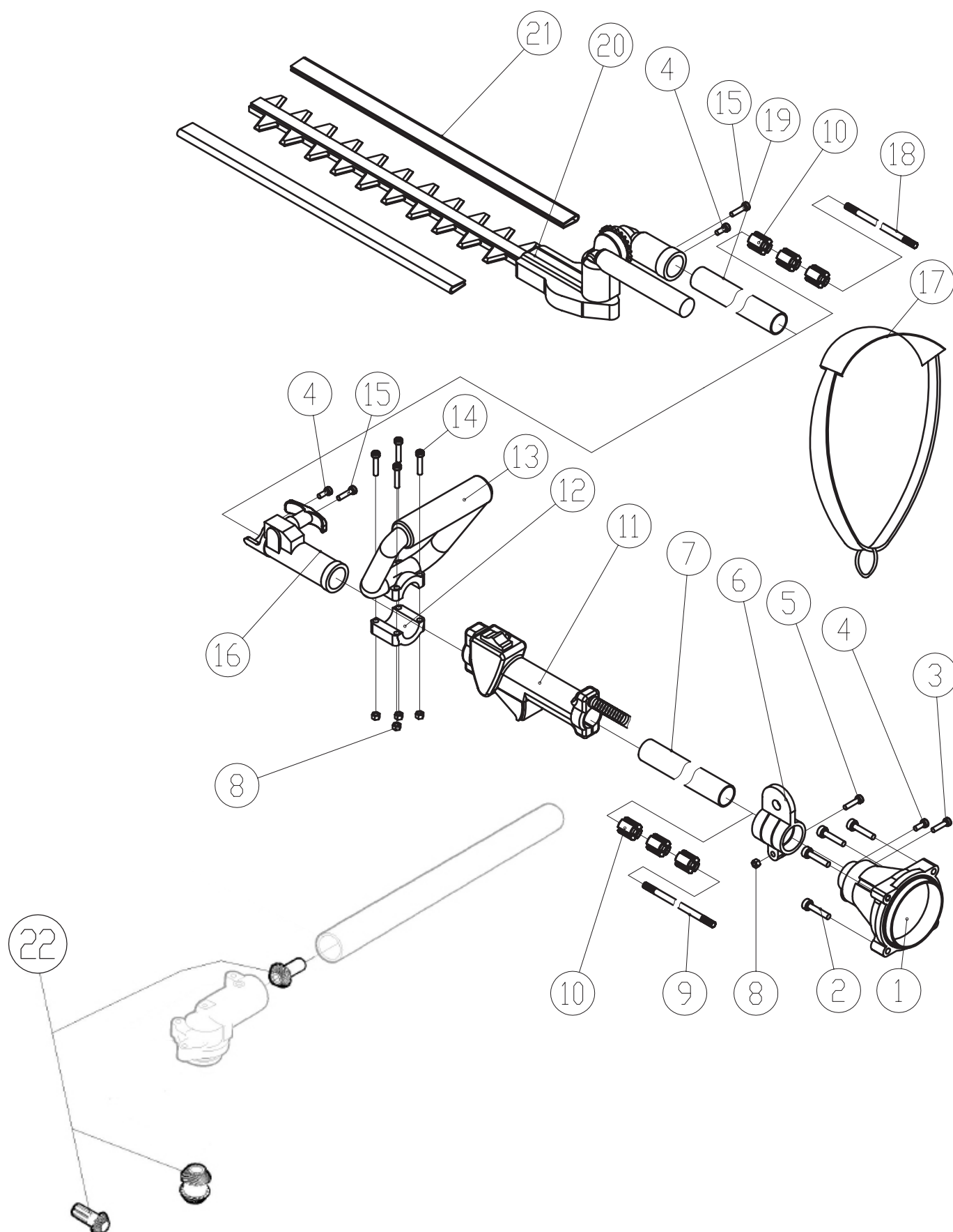
FIGURA 2: PARTE DEL CORTASETOS
